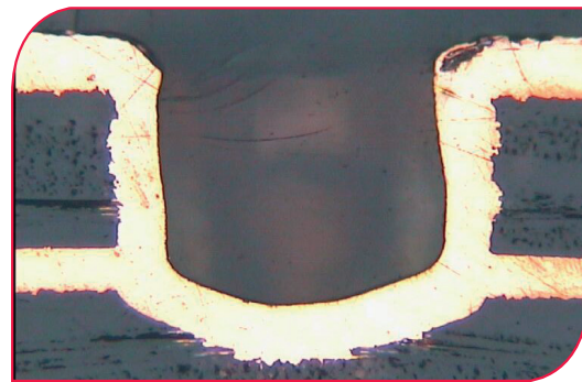
Blind Via mit Standardwerkzeug
